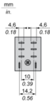
Vue côté broches
