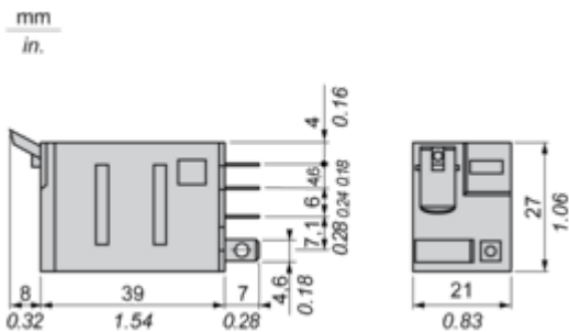
Vue côté broches
